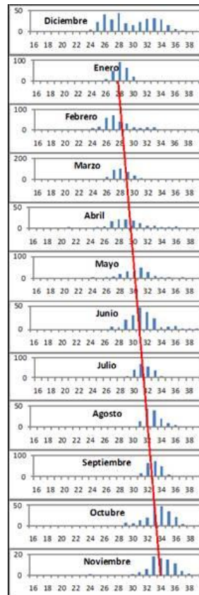
Figura 13: Distribución de frecuencias por talla para Hemiramphus saltator muestreado en el Golfo Dulce y en el periodo diciembre 2009 a noviembre 2010.
